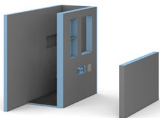
Moduldusche und angebundene Modulwand Kombination aus praktischen Nischen, technischen Vorfertigungen und angebundener Trennwand
