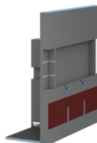
Dreiseitig genutztes T-Modul Systemlösung für WC, Dusche und Waschbecken inkl. technischer Komponenten und Verstärkungen
